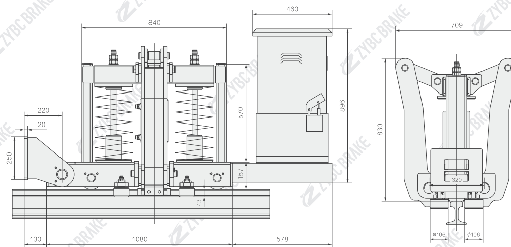
型号 Type: ZYTJX-250
