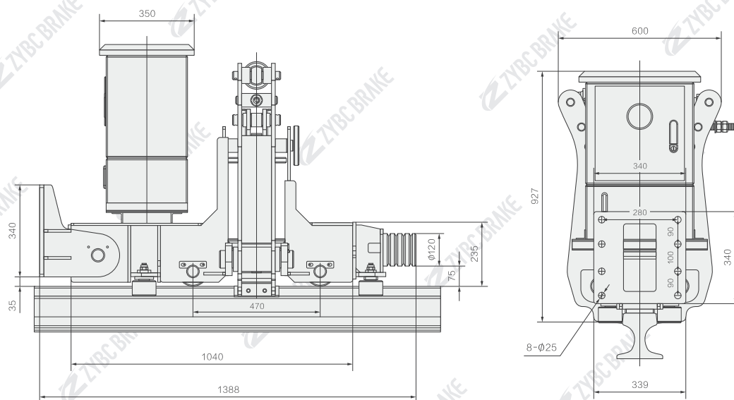
型号 Type: ZYTJX-120
